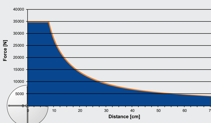
Max rotation torque 2800 Nm
